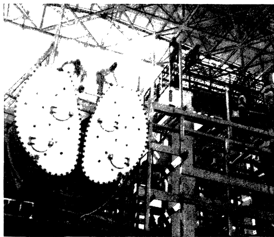
Монтаж конденсатора электростанции «Мариель». 1964.
